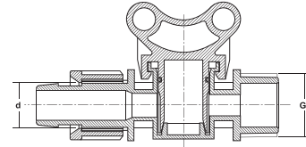
MİNİ VANA DAMLAMA - ERKEK MINI VALVE DRIPLINE - MALE МИНИ КРАН (СИНИЙ) ДЛЯ КАПЕЛЬНЫХ ТРУБОК - РЕЗЬБА سکر ذکر - راکور
