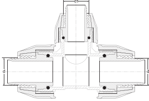
REDÜKSİYON TE REDUCING TEE
