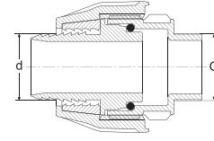
ERKEK ADAPTÖR MALE ADAPTOR
