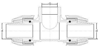
DIŞİ TE FEMALE TEE
