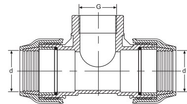
KABLİN DIŞİ TE FEMALE TEE ТРОЙНИК С ВНУТРЕН.РЕ.З. تی خرطوم سن داخلی
