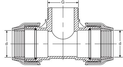
KABLİN ERKEK TE MALE TEE ТРОЙНИК С НАРУЖН.РЕ.З. تی خرطوم سن خارجی
